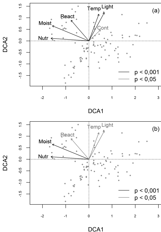
Obr. 1. – Ordinační diagram detrendované korespondenční analýzy (DCA) s pasivně proloženými průměrnými Ellenbergovými indikačními hodnotami pro světlo (Light), teplotu (Temp), kontinentalitu (Cont), vlhkost (Moist), živiny (Nutr) a půdní reakci (React). Míra průkaznosti vztahu průměrných EIIV k ordinačním osám je vyjádřena následovně: černé vektory zobrazují proměnné průkazné na hladině p < 0,001 , šedé na p < 0,05 , neprůkazné proměnné nejsou zobrazeny. Pro hodnoty průkaznosti viz tab. 1. (a) Průkaznost počítána původním permutačním testem, (b) průkaznost počítána modifikovaným permutačním testem. Body v diagramu zobrazují pozice jednotlivých vegetačních zápisů.
