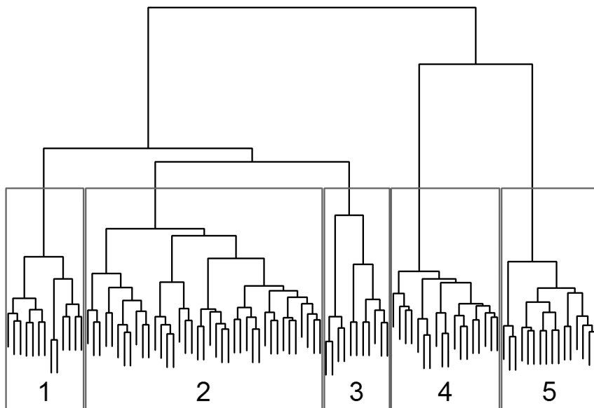
Obr. 4. – Dendrogram shlukové analýzy, která rozdělila vegetační zápisy z údolí Vltavy do pěti vegetačních typů, ohraničených šedými obdélníky s číslem vegetačního typu. Čísla vegetačních typů jsou vysvětlena v popisku k obr. 5.
