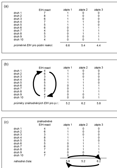
Obr. 2. – Schematické znázornění výpočtu (a) průměrných Ellenbergových indikačních hodnot pro půdní reakci, (b) průměrů znáhodněných EIH pro půdní reakci a (c) náhodných čísel . Pro podrobnosti výpočtu viz hlavní text.
